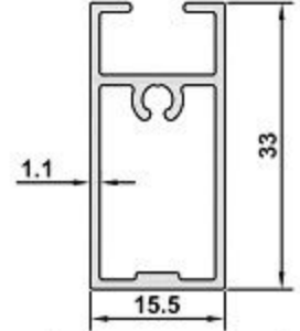
3205 AĞIRLIK / WEIGHT 0,342 kg/m
