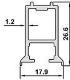
3206 AĞIRLIK / WEIGHT 0,295 kg/m
