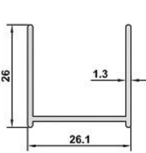
DK-57 AĞIRLIK / WEIGHT 0,266 kg/m
