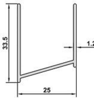
DK-62 AĞIRLIK / WEIGHT 0,271 kg/m
