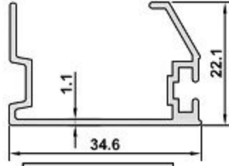
DK-52 AĞIRLIK / WEIGHT 0,298 kg/m
