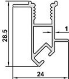
DK-65 AĞIRLIK / WEIGHT 0,276 kg/m
