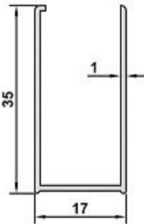
2555 AĞIRLIK / WEIGHT 0,230 kg/m
