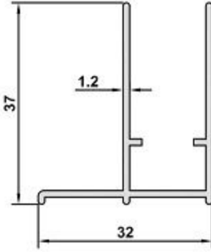
3202 AĞIRLIK / WEIGHT 0,352 kg/m
