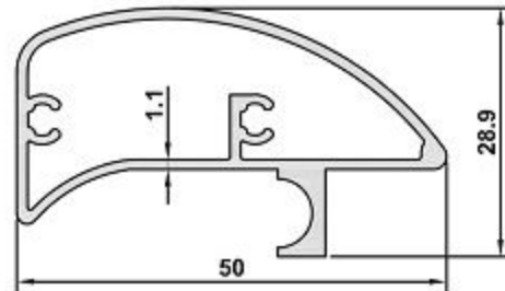
DK-13 AĞIRLIK / WEIGHT 0,575 kg/m
