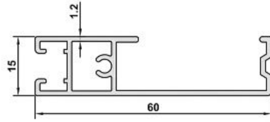
3210 AĞIRLIK / WEIGHT 0,493 kg/m
