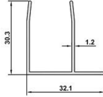
DK-15 AĞIRLIK / WEIGHT 0,282 kg/m
