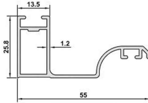
DK-06 AĞIRLIK / WEIGHT 0,461 kg/m
