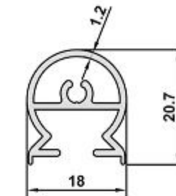
3209 AĞIRLIK / WEIGHT 0,279 kg/m
