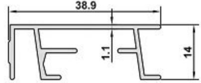
2558 AĞIRLIK / WEIGHT 0,306 kg/m
