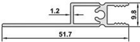
DK-55 AĞIRLIK / WEIGHT 0,317 kg/m
