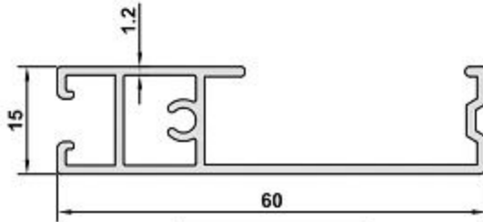
3217 AĞIRLIK / WEIGHT 0,488 kg/m
