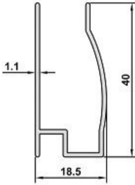
DK-24 AĞIRLIK / WEIGHT 0,303 kg/m
