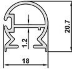
3203 AĞIRLIK / WEIGHT 0,263 kg/m
