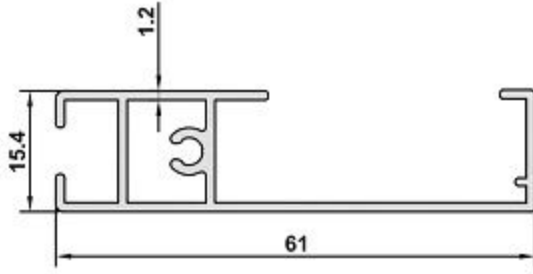
DK-07 AĞIRLIK / WEIGHT 0,472 kg/m
