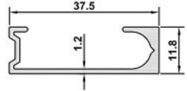
6464 AĞIRLIK / WEIGHT 0,280 kg/m
