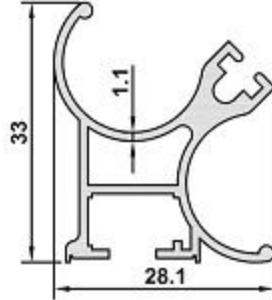
DK-05 AĞIRLIK / WEIGHT 0,436 kg/m
