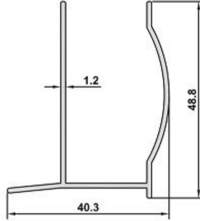
DK-18 AĞIRLIK / WEIGHT 0,423 kg/m
