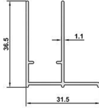
DK-09 AĞIRLIK / WEIGHT 0,317 kg/m
