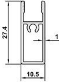
DK-61 AĞIRLIK / WEIGHT 0,231 kg/m
