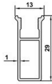
DK-54 AĞIRLIK / WEIGHT 0,222 kg/m
