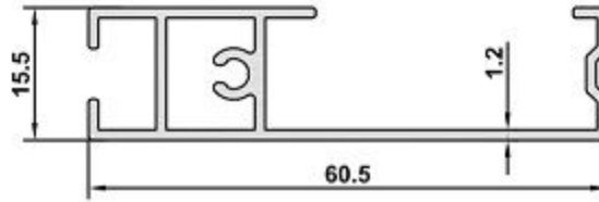
DK-08 AĞIRLIK / WEIGHT 0,491 kg/m
