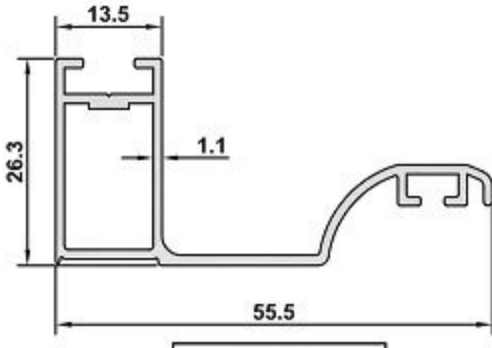
3212 AĞIRLIK / WEIGHT 0,456 kg/m
