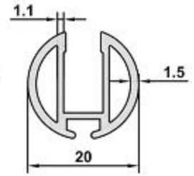
DK-21 AĞIRLIK / WEIGHT 0,315 kg/m
