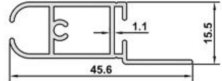
2553 AĞIRLIK / WEIGHT 0,350 kg/m
