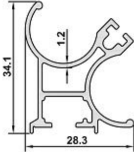
3207 AĞIRLIK / WEIGHT 0,412 kg/m
