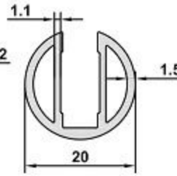
DK-20 AĞIRLIK / WEIGHT 0,317 kg/m
