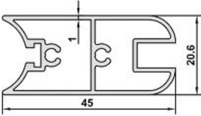
DK-19 AĞIRLIK / WEIGHT 0,566 kg/m
