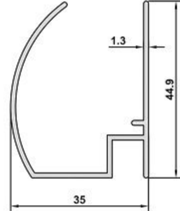
DK-14 AĞIRLIK / WEIGHT 0,455 kg/m
