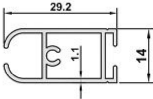
2552 AĞIRLIK / WEIGHT 0,298 kg/m
