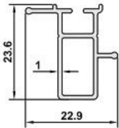
DK-63 AĞIRLIK / WEIGHT 0,222 kg/φ
