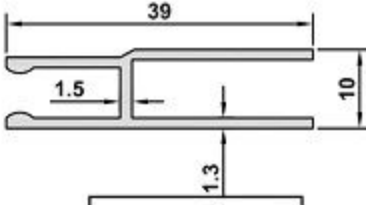
4670 AĞIRLIK / WEIGHT 0,312 kg/m
