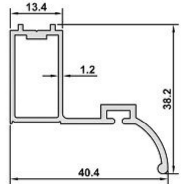
3200 AĞIRLIK / WEIGHT 0,442 kg/m
