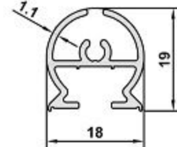
DK-17 AĞIRLIK / WEIGHT 0,239 kg/m
