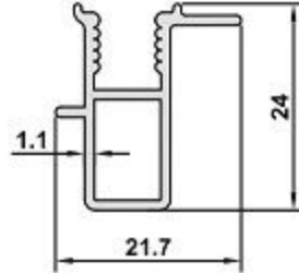
DK-51 AĞIRLIK / WEIGHT 0,252 kg/m
