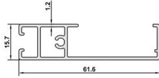
3211 AĞIRLIK / WEIGHT 0,496 kg/m
