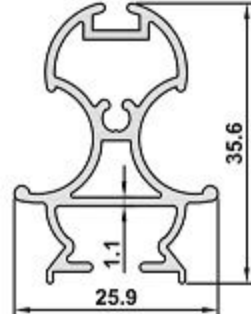
3204 AĞIRLIK / WEIGHT 0,455 kg/m
