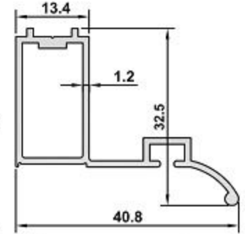
DK-11 AĞIRLIK / WEIGHT 0,380 kg/m
