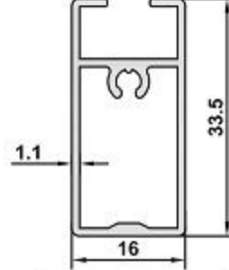
DK-04 AĞIRLIK / WEIGHT 0,347 kg/m
