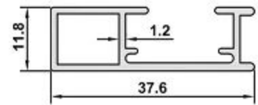
3213 AĞIRLIK / WEIGHT 0,331 kg/m
