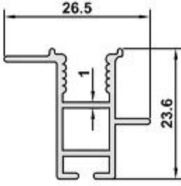
DK-64 AĞIRLIK / WEIGHT 0,268 kg/m
