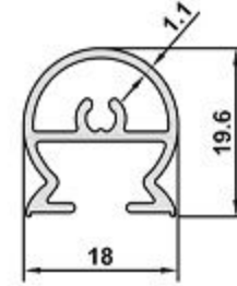
DK-02 AĞIRLIK / WEIGHT 0,255 kg/m
